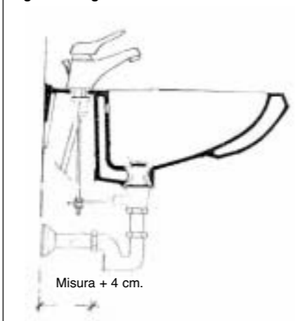
Fig. 5 - Collegamento canotto
