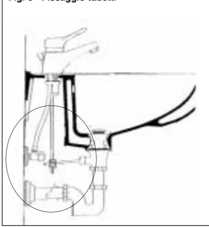
Fig. 6 - Fissaggio tubetti
