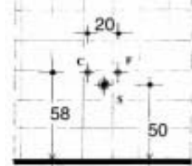
Fig. 2 - Montaggio rubinetto
