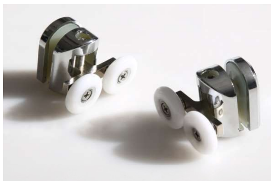
Cuscinetti doppi superiori con supporto in ABS cromato
